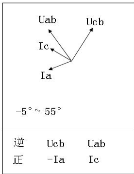
A、C相电压接反
